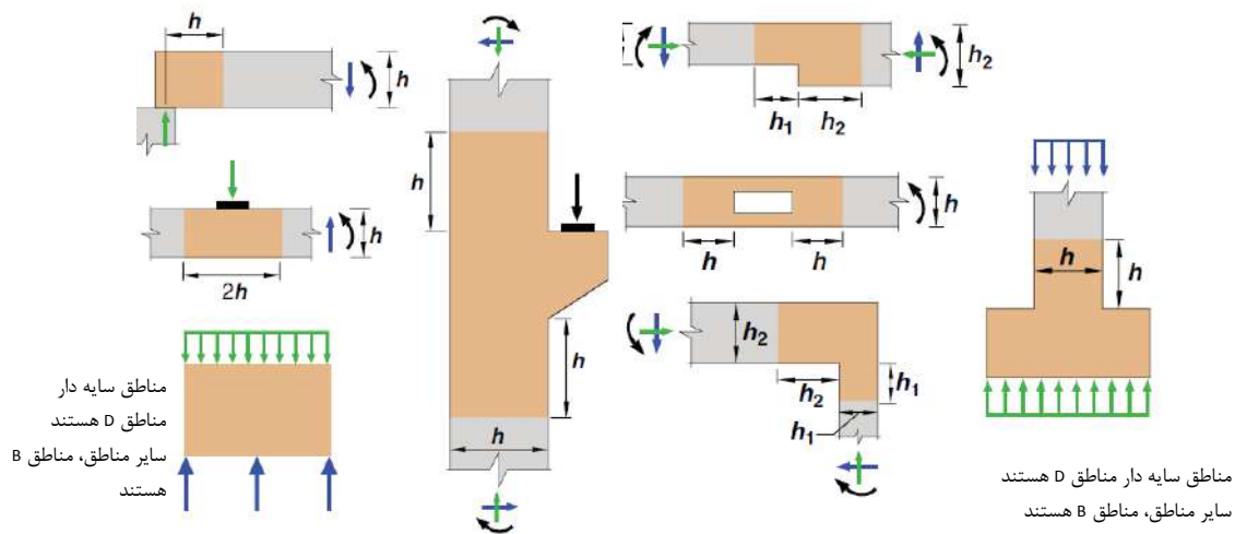
شکل ۱-۲۲ ناپیوستگی هندسی
