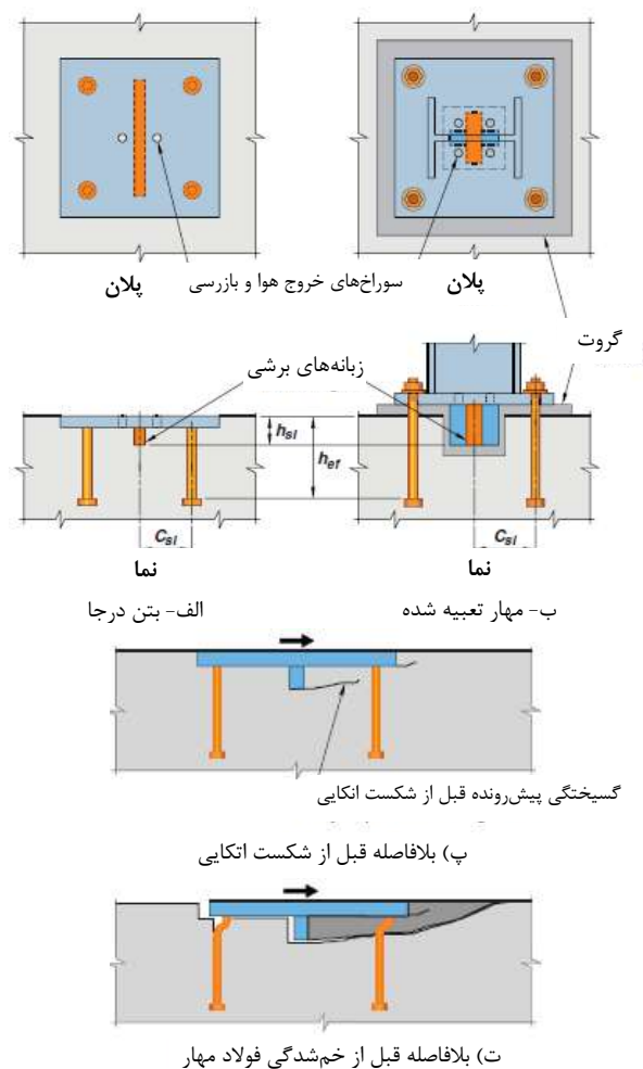
شکل ۱۱-۱۸ شکست اتکایی و خم‌شدگی مهار برای صفحه جاگذاری شده زبانه برشی
