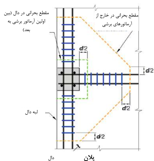
شکل ۳-۸ ب مقاطع بحرانی برش دوطرفه در دال با آرماتور برشی پیرامون یک ستون کناری
