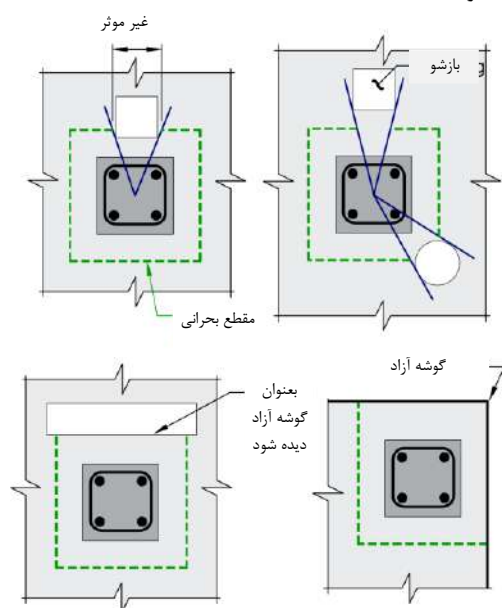
شکل ۴-۸ تاثیر بازشو و لبه‌های آزاد بر مقطع بحرانی (توجه: بازشوها در محدوده 4h از محیط ستون فرض شده‌اند).
