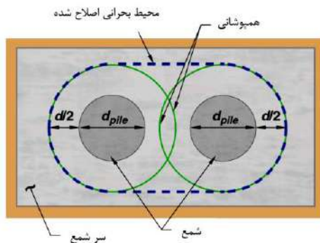
شکل ۳-۱۵ محیط بحرانی اصلاح شده برای برش در محدوده‌های بحرانی دارای همپوشانی
