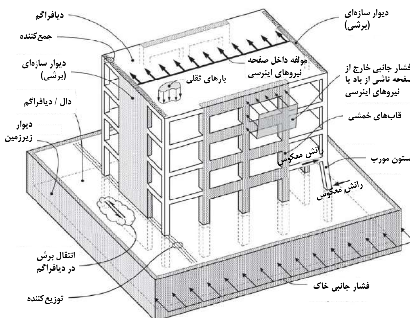
شکل ۱-۱۴ نیروهای وارد بر دیافراگم
