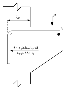
شکل ۲-۱۷ نمونه مهار در دو انتهای آرماتور اصلی
