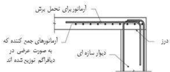
شکل ۵-۱۴ جزئیات شماتیک عملکرد شاخه‌ای آرماتور که برای انتقال برش به دیوار سازه‌ای از طریق برش اصطکاکی تامین شده‌است.
