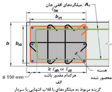
شکل ۱۷-۲۰ گیرایی آرماتور افقی یا خم‌دار دیوار در بتن محصور شده
