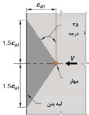
پلان
