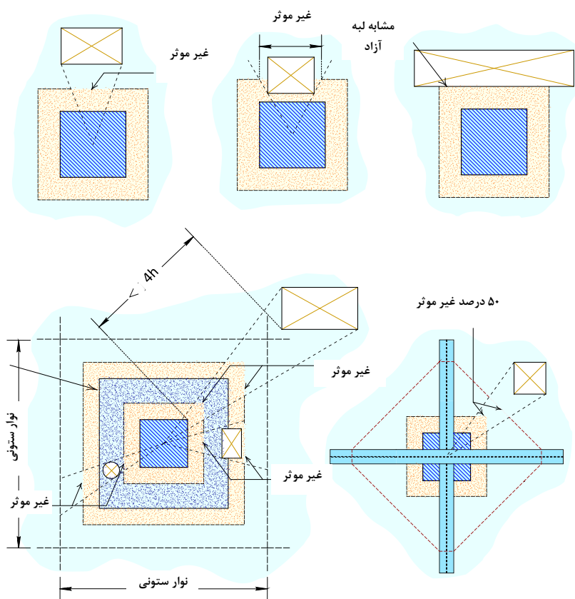
شکل ۸-۲ تأثیر بازشو در دال بر سطح موثر مقطع بحرانی
