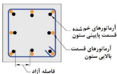
شکل ۲-۱۲ آرماتورهای خم شده ستون
