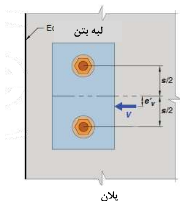
شکل ۹-۱۸ تعریف e'_v برای گروه مهار
