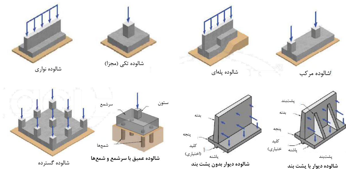
شکل ۱۵-۱ بعضی از انواع شالوده‌ها
