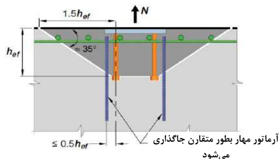
مقطع A-A
