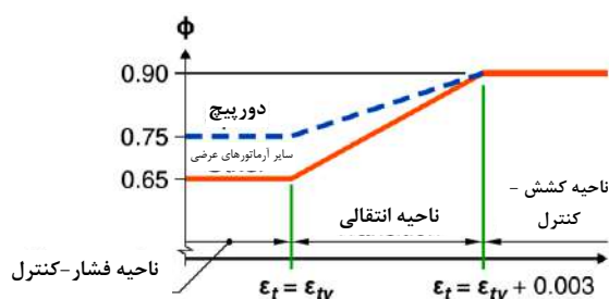
شکل ۲-۷ تغییرات \phi بر اساس کرنش کششی خالص در دورترین فولاد کششی
