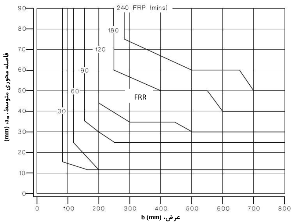
شکل ۲۳-۴ مدت زمان مقاومت در برابر آتش برای تیرهای پیوسته
