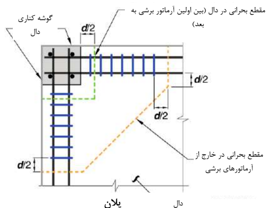
شکل ۳-۸ پ مقاطع بحرانی برش دوطرفه در دال با آرماتور برشی پیرامون یک ستون گوشه
