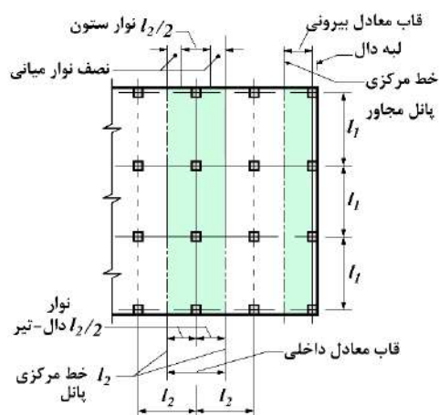
شکل ۱۱-۱۰ تعریف قاب معادل
