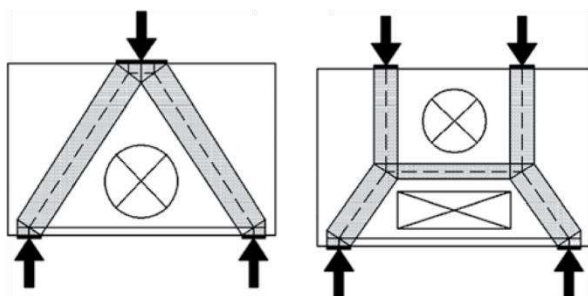
شکل ۲۲-۸ تعیین محل‌های مناسب ایجاد بازشو در تیرهای عمیق
