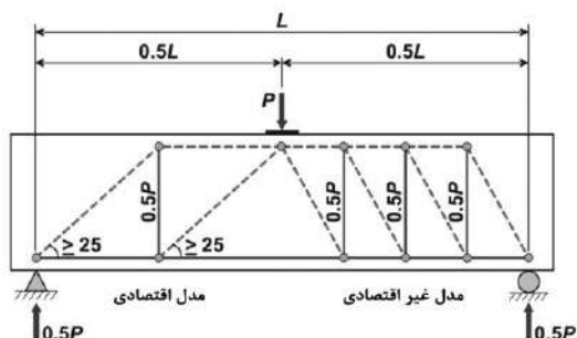
شکل ۲۲-۷ مدل‌های خرابایی انتخابی اقتصادی و غیر اقتصادی
