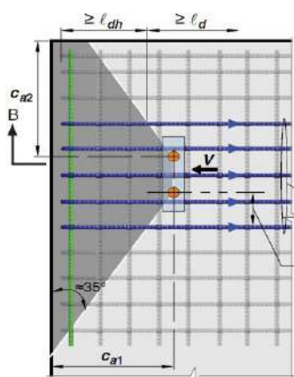
پلان
