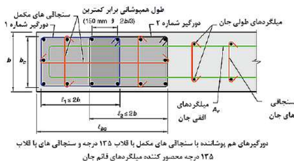
شکل ۲۰-۱۸ شکل آرماتورهای عرضی جز مرزی و سنگجایی های جان
