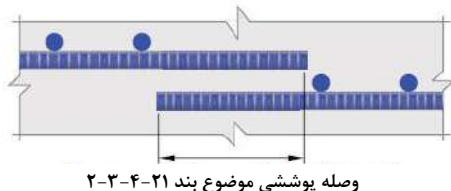
شکل ۲۱-۹ وصله پوششی شبکه سیم‌های آجدار جوش‌شده
