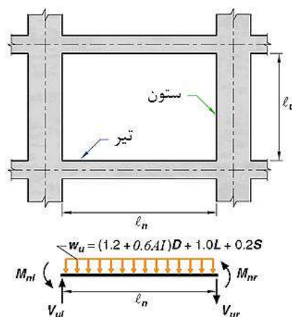
شکل ۲۰-۲ محاسبه برش در تیرها (روش مقاومتی)
