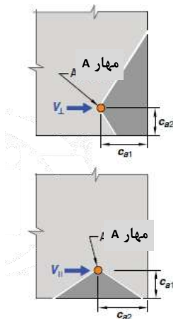
ت- نیروی برشی نزدیک یک گوشه
