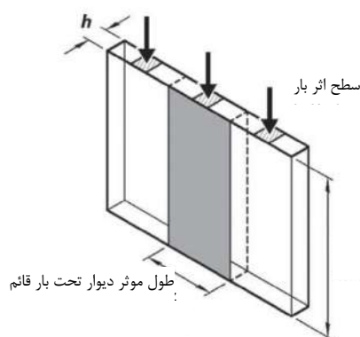
شکل ۱-۱۳ عرض موثر دیوار تحت بارهای متمرکز
