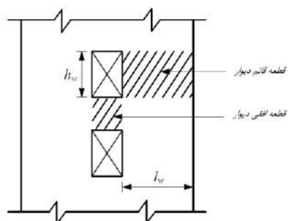
شکل ۲۰-۱۰ دیوار سازه‌ای با بازشو
