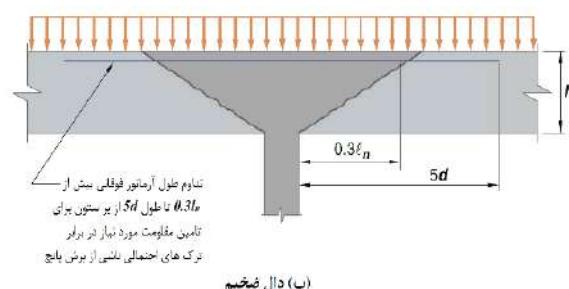
شکل ۶-۱۰ ترک‌های ناشی از برش دوطرفه در دال‌های معمولی و ضخیم
