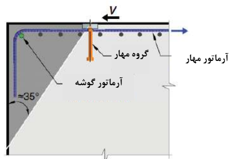
(ب) آرماتور مهار سنجاقی برای مهار برش
