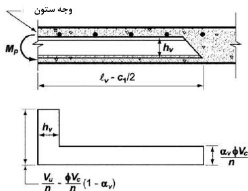
شکل ۸-۷ برش ایده‌آل در کلاhek برشی
