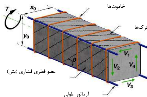
شکل ۸-۱۱ الف تشابه خریای فضایی
