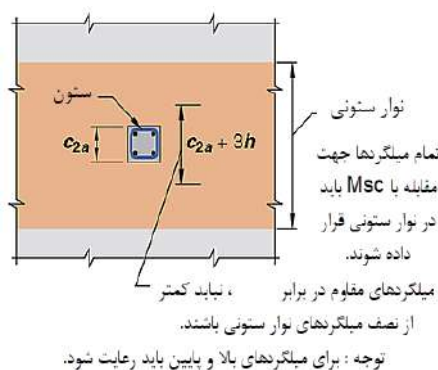
شکل ۲۰-۴-الف عرض موثر دال در ستون‌های میانی
