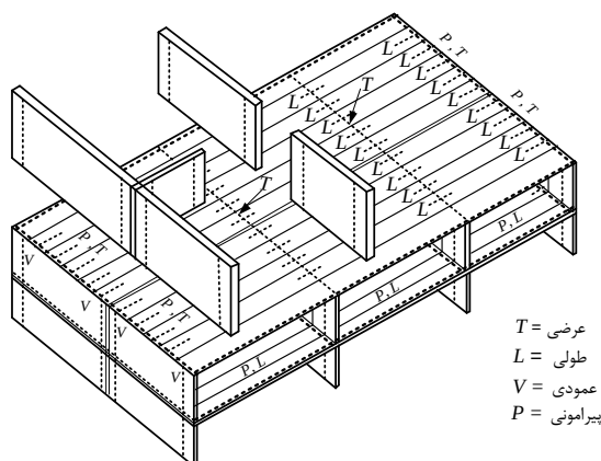
شکل ۴-۱۷ آرایش متداول کلاف‌های انسجام در سازه‌های با ارتفاع سه طبقه و بیشتر
