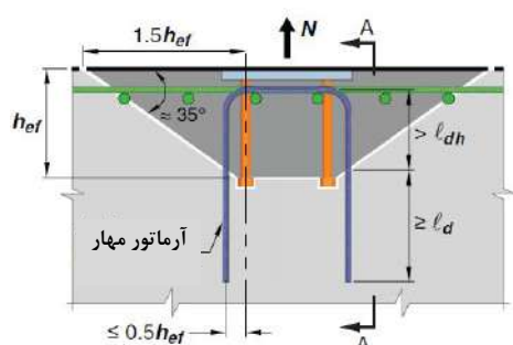
نما
