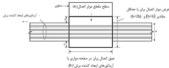
برش افقی اتصال
