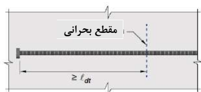
الف- طول گیرایی میلگرد آجدار سردار
