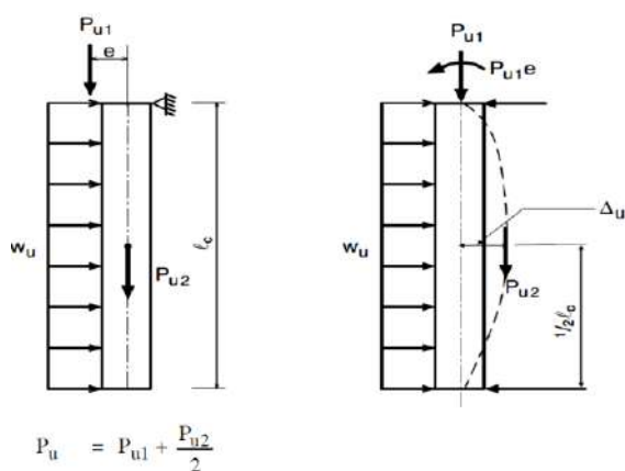
شکل ۴-۱۳ مدل دیوار در تحلیل خارج از صفحه دیوارهای لاغر به روش جایگزین
