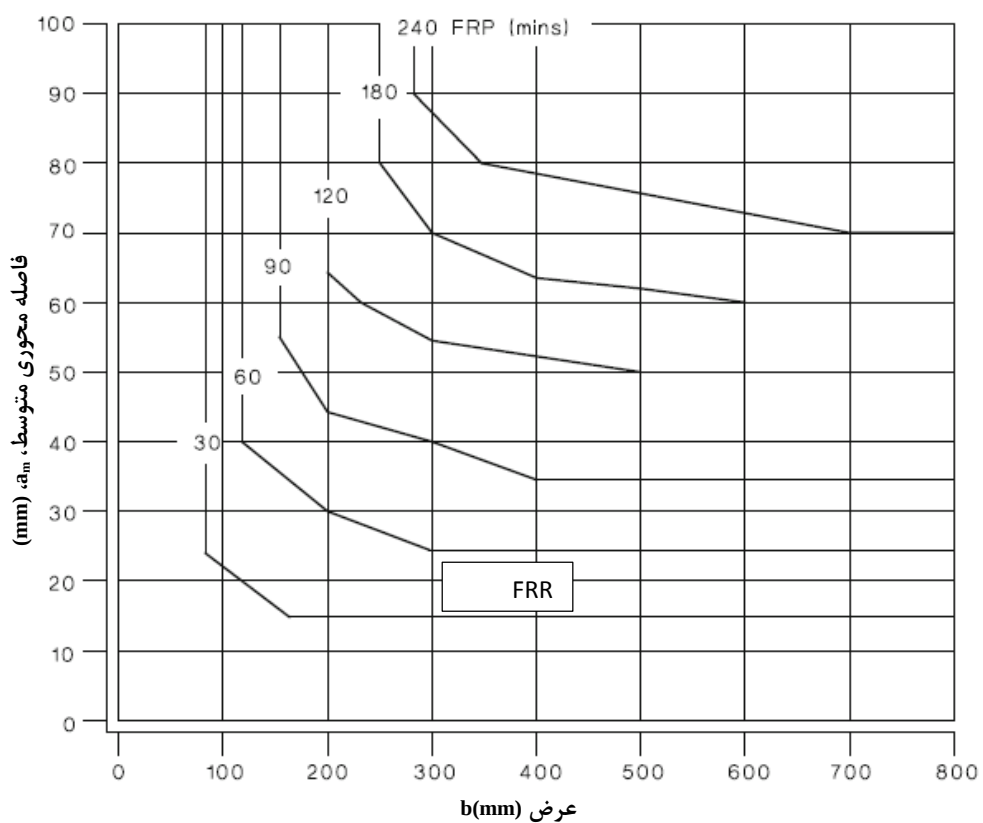
شکل ۲۳-۳ مدت زمان مقاومت در برابر آتش برای تیرهای ساده
