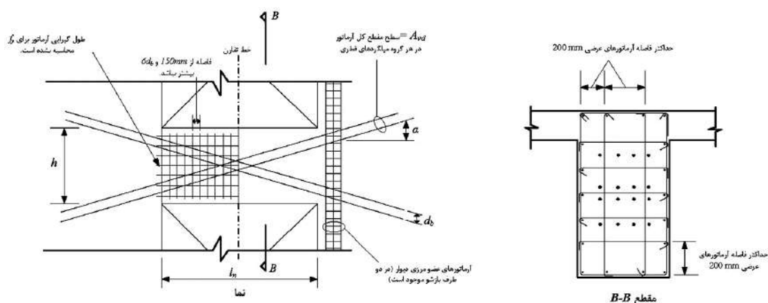
ب - محصور شدگی کلی هر دو گروه آرماتورهای قطری
