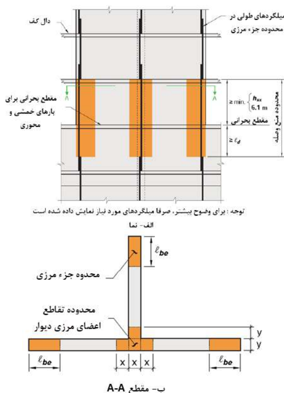
شکل ۲۰-۱۴ اجزا مرزی دیوارها در ارتفاع که در آن‌ها وصله‌های پوششی مجاز نیست
