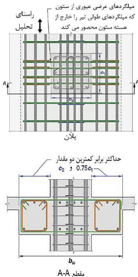
شکل ۵-۲۰ حداکثر عرض موثر در تیرهای پهن و آرمانور عرضی مورد نیاز
