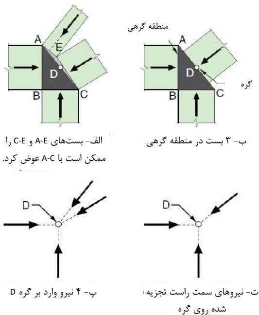
شکل ۲۲-۴ تجزیه نیروهای وارد به منطقه گرهی
