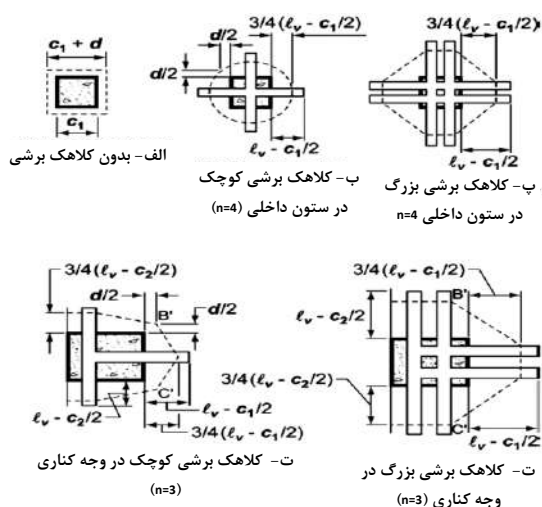
شکل ۸-۸ موقعیت مقطع بحرانی در کلاهک برشی
