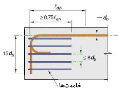
(الف) آرماتور محصور کننده بموازات آرماتور اصلی
