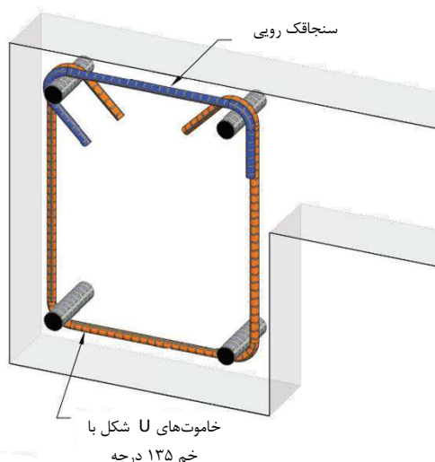
شکل ۱۱-۷ مثالی از خاموت دو تکه که با ضوابط بند ۱۱-۶-۵ خوانایی دارد
