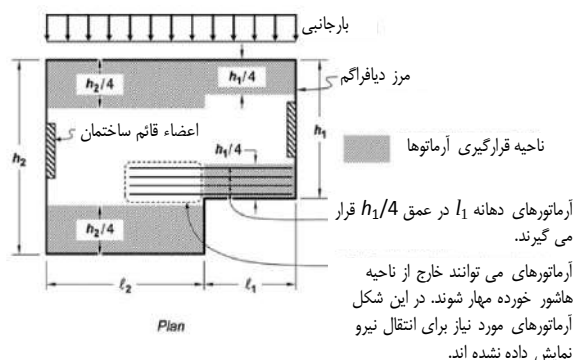
شکل ۴-۱۴ موقعیت آرماتورهای غیرپیش‌تنیده که در برابر نیروی کششی ناشی از خمش و نیروی محوری مقاومت می‌کنند.
