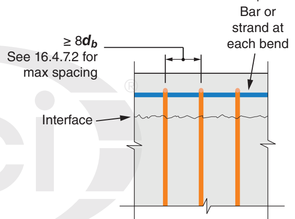
b) Longitudinal Section
