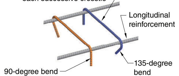
Fig. R25.3.5—Crosstie.
